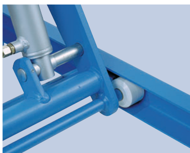
| Scherenrollen in der Unterrahmenkonstruktion
